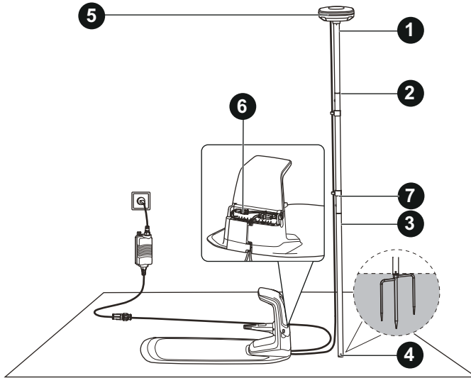
אפשרות 1: הטענת אנטנת הייחוס באמצעות עמדת הטעינה
