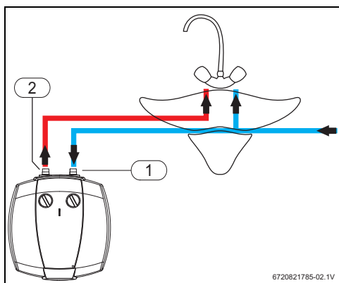
8. ábra Mosdókagyló alatt történő szerelés
