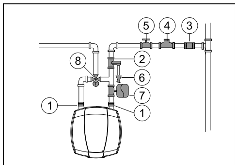
10. ábra Vízbekötés
