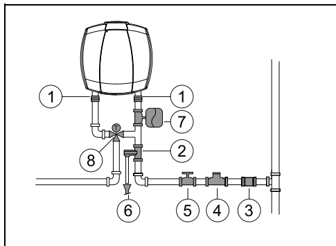
9. ábra Vízbekötés
