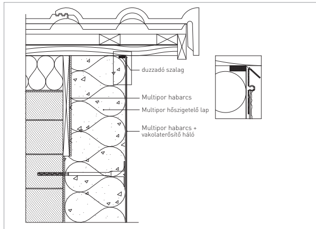
Ereszcsatlakozás 1.
