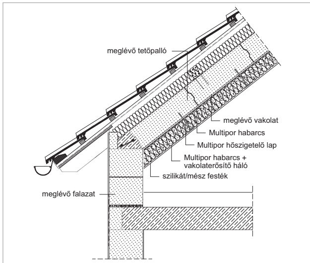
Tetőtér, pallófödém 1.
