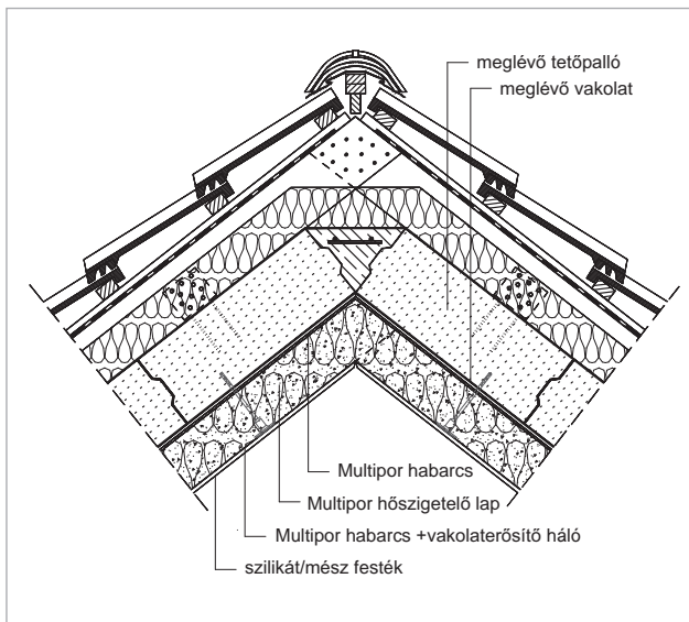
Tetőtér pallófödém 3.
