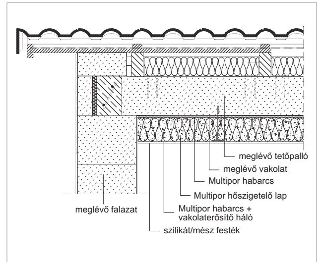
Tetőtér pallófödém 2.
