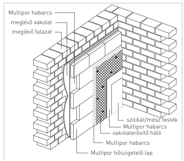
Rétegrend
