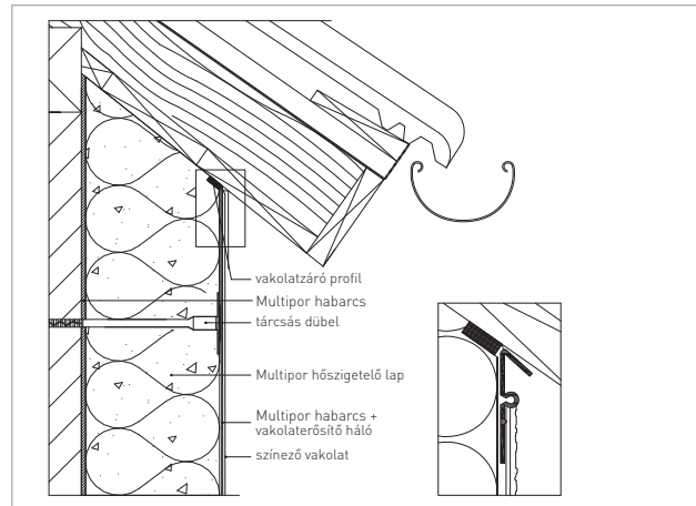
Ereszcsatlakozás 2.
