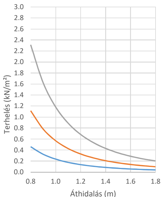
Terhelés/ Áthidalás
